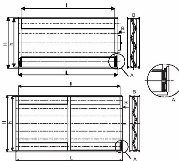
МОНТАЖ В СТЕНЕ
